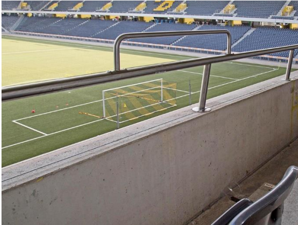
Abbildung 46 Absturzicherung bei Stehplätzen
