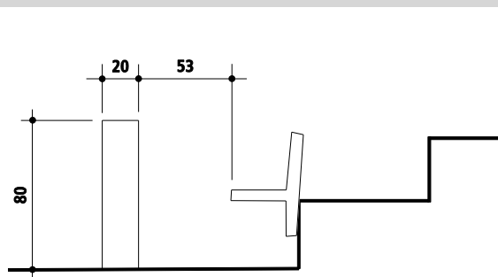
Abbildung 44 Absperrungen auf gleicher Ebene
