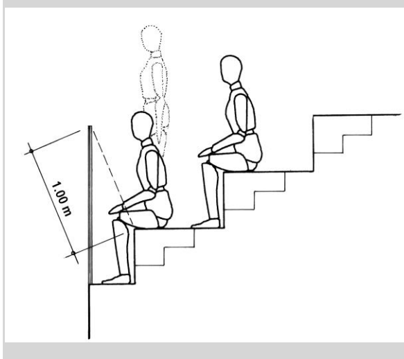
Abbildung 47 Absturzicherung bei Sitzplätzen, Beispiel A
