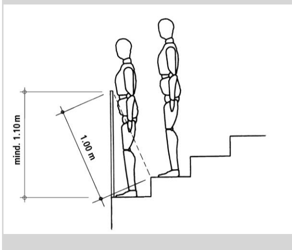
Abbildung 47 Absturzicherung bei Sitzplätzen, Beispiel A
