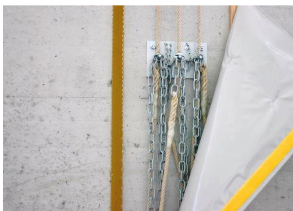
Abbildung 17 Nachträglich montierte Abdeckung mit Klettverschluss befestigt
