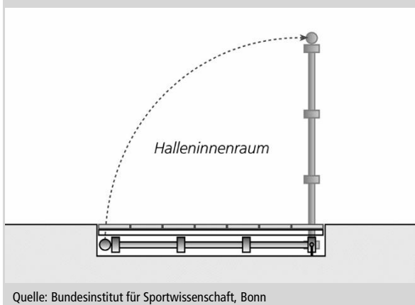
Abbildung 15 Schematische Darstellung eines wandbündigen Abschlusses einer Gerätenische für eine schwenkbare Sprossenwand
