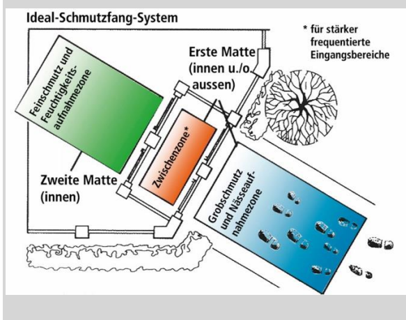
Abbildung 1 Schema eines fachgerechten Schmutzschleusensystems
