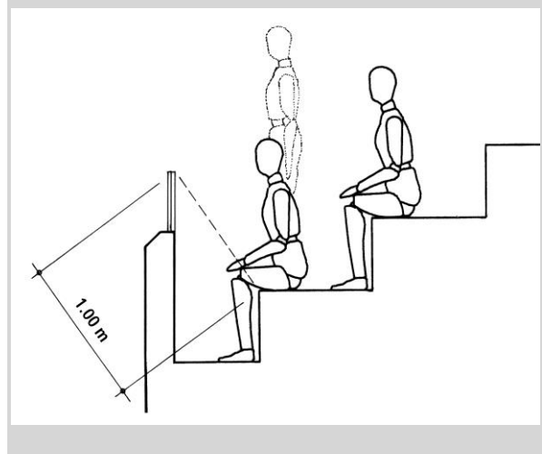
Abbildung 50 Absturzicherung bei Sitzplätzen, Beispiel C
